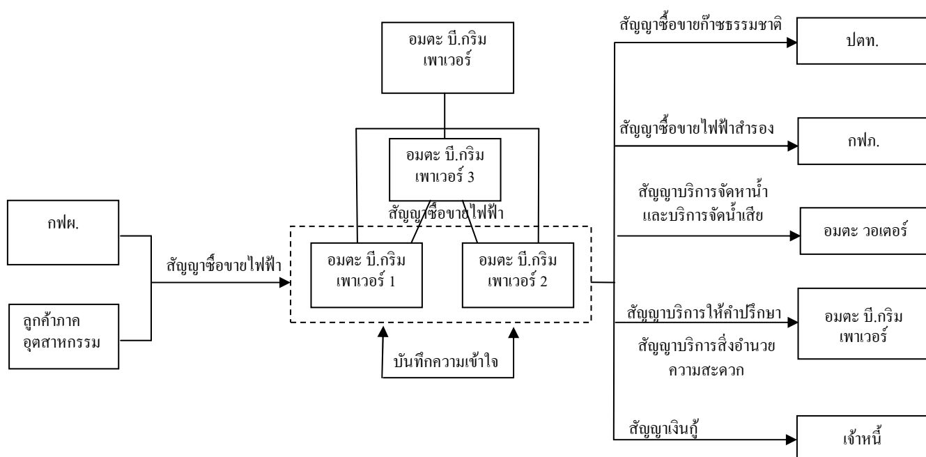
แผนภาพที่ 4-3: แผนภาพโครงสร้างพื้นที่เกี่ยวข้องกับปี.กริม 1 และปี.กริม 2
