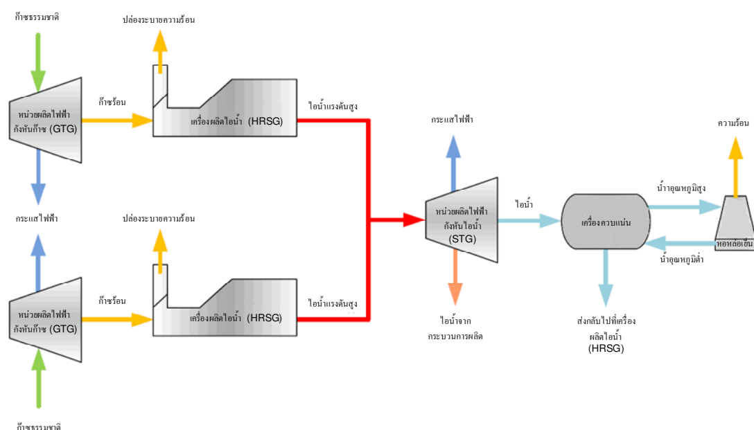
รูปภาพที่ 4-1: กระบวนการผลิตไฟฟ้าพลังความร้อนร่วม
